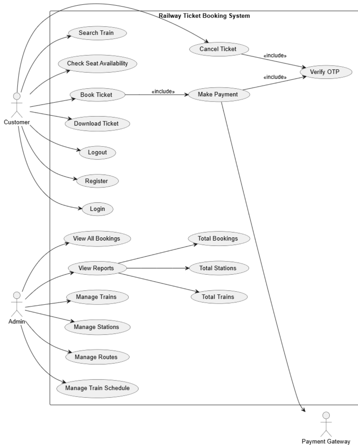
Fig 1 : UseCase Diagram
